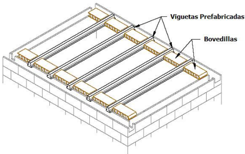
Figura 1 – Colocación de las Viguetas No se ha dibujado el apuntalado
