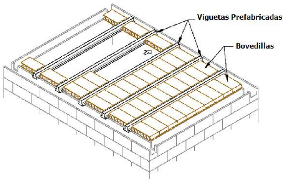
Figura 2 – Colocación de las Bovedillas
